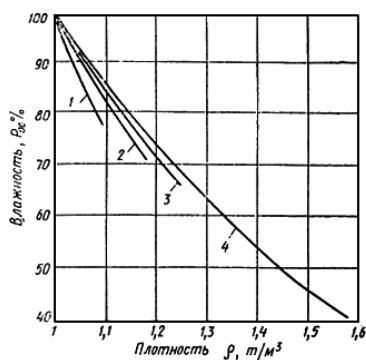
Рис.5. Значения плотности в зависимости от влажности осадка станций осветления и обезжелезивания воды
