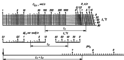
Рис.1. Номограмма для определения pH насыщения воды карбонатом кальция ( \text{pH}_s )
